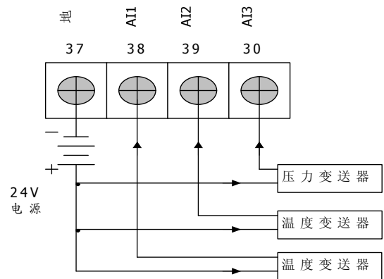
模拟输入接线示意图
