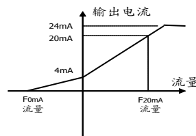
0-4-20mA 方式输出特性
