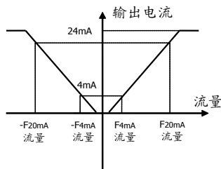
20-4-20mA 方式输出特性
