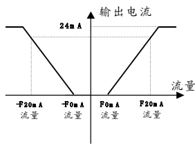
20-0-20mA 方式输出特性
