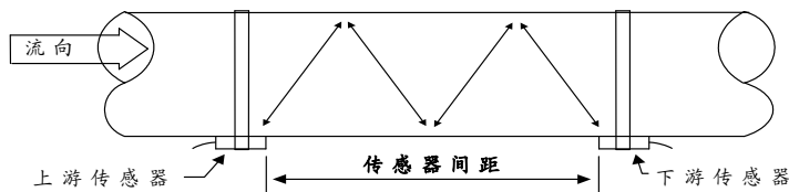
W 法 — 顶视图
