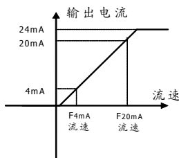
流速 4-20mA 方式输出特性
