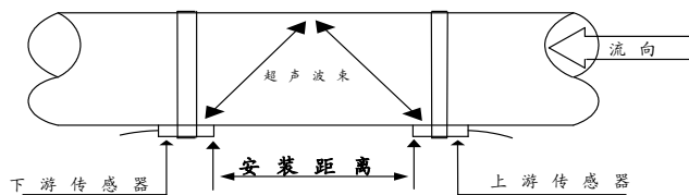
V 法 — 顶视图
