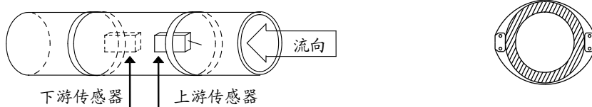
Z 法 — 侧视图
