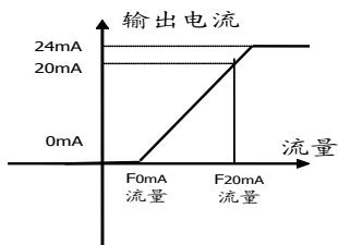
0-20mA 方式输出特性
